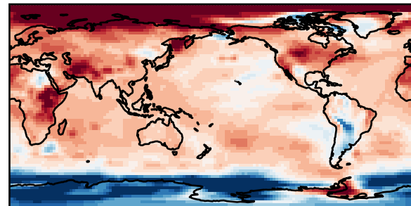
20CR
