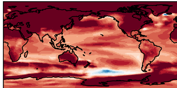
MIROC-ESM
